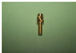
BSF147P QTY: 12 Insonic stud M4 x 10mm BR SC
